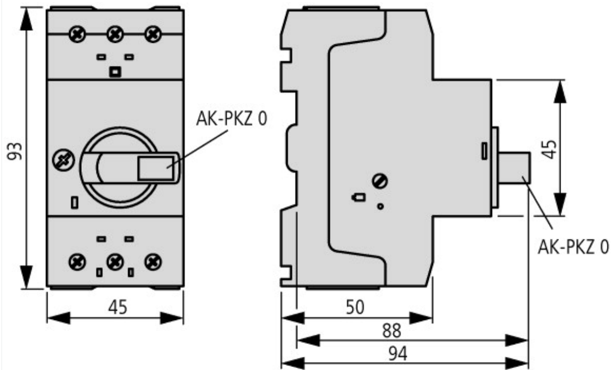
Motorschutzschalter mit abschließbarem Drehknebel PKZM0-...+AK-PKZ0
